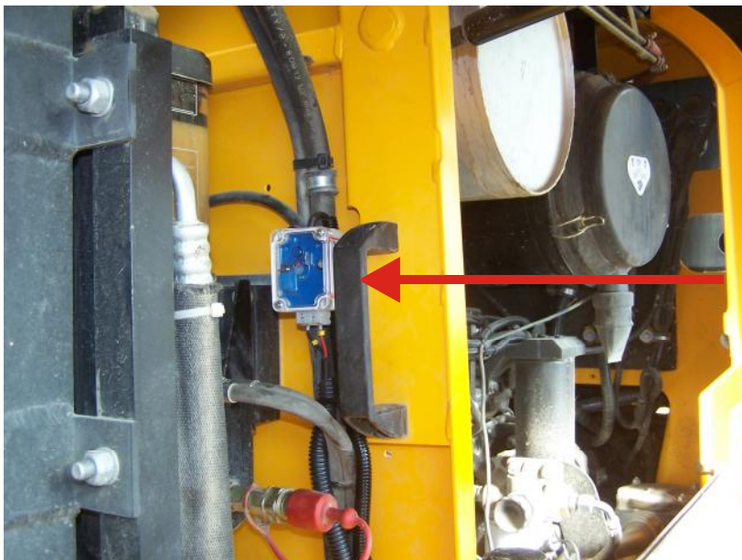
Installation des elektronischen Modulators an der Motorschottwand
