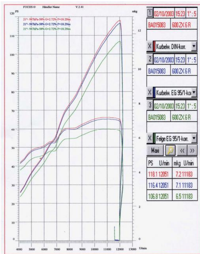
Leistungsmessbericht ohne AIR-TEC
