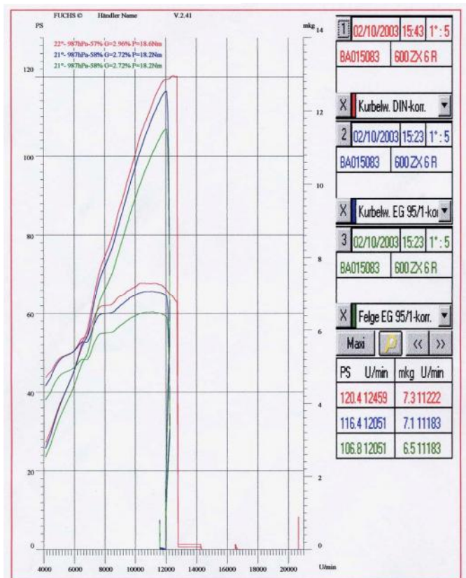
Leistungsmessbericht mit AIR-TEC
